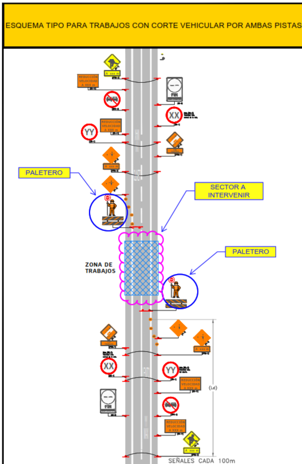
Figura 1: Esquema para trabajos con corte vehicular por ambas pistas.
