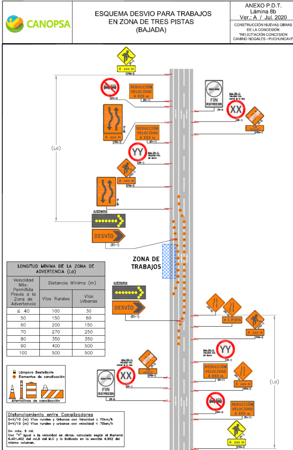
Figura 2: Esquema desvío para trabajos en zona de 3 (bajada)
