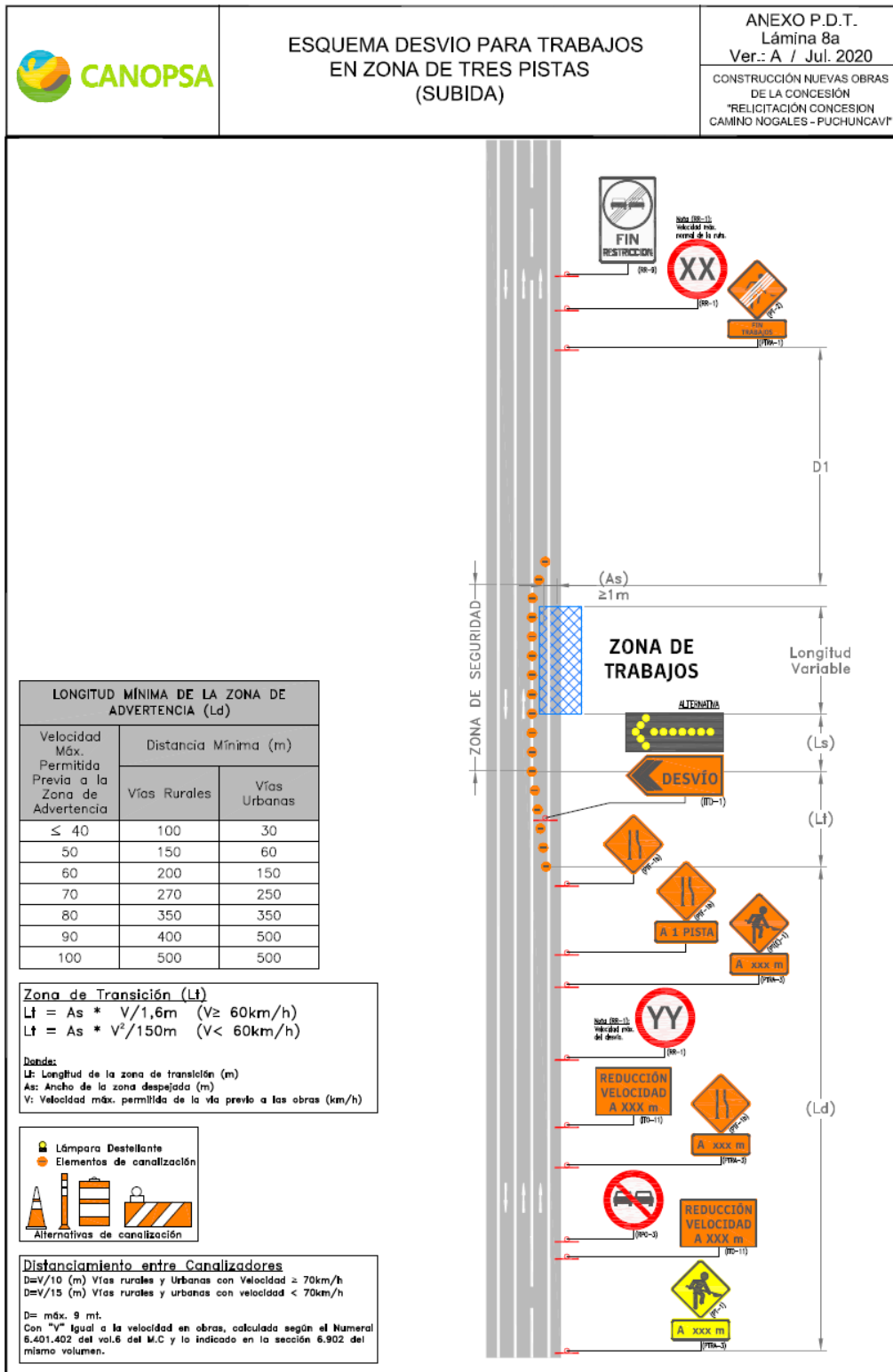
Figura 1: Esquema desvío para trabajos en zona de 3 pistas (subida)
