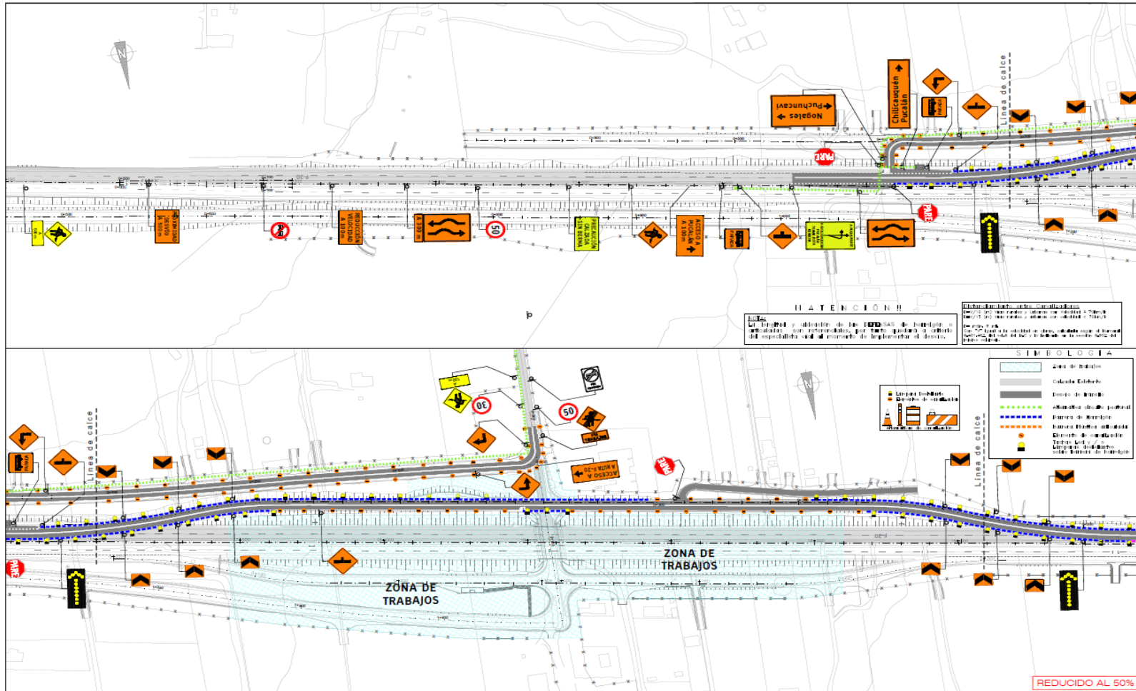
Figura 1: Planos emplazamiento gestión de tráfico de contingencia Pucalán 2
