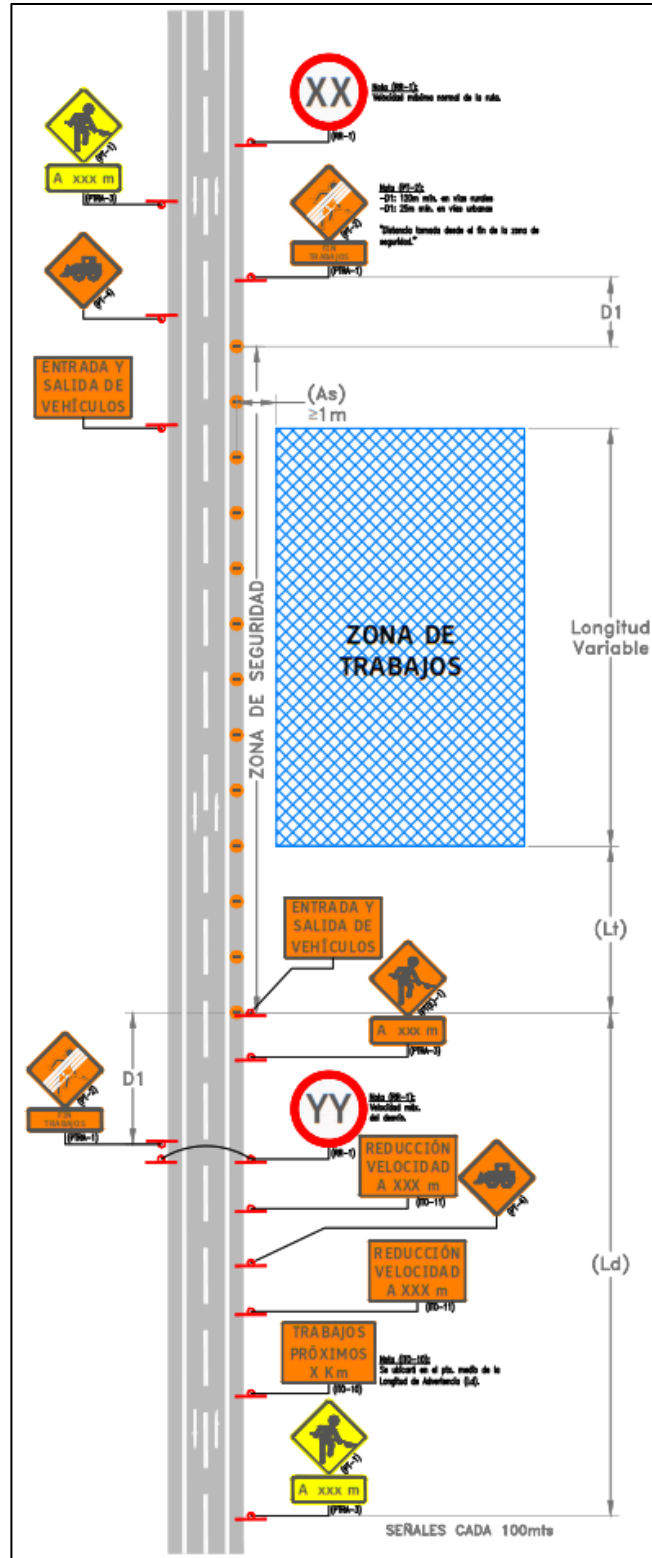
Figura 1: Esquema gestión de tráfico para trabajos.
