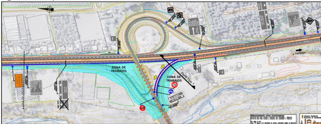
Figura 1: Esquema Fase 3 Gestión de Tráfico sector Enlace Ruta-5
